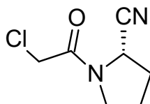
(2S)-1-(Chloroacetyl)-2-pyrrolidinecarbonitrile
